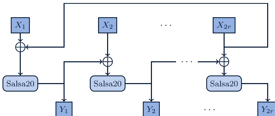
Figura 2 - Algoritmo BlockMix interno a script
